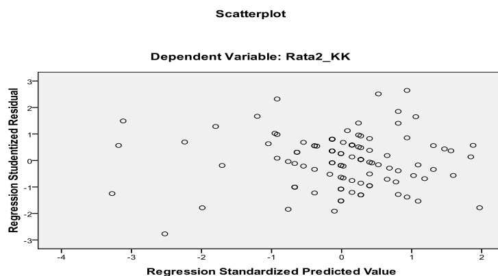
Gambar 3 Grafik Scatterplot
