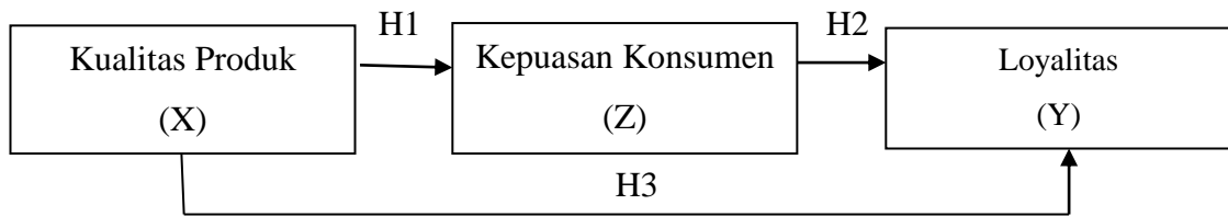
Gambar 1. Kerangka Konseptual
